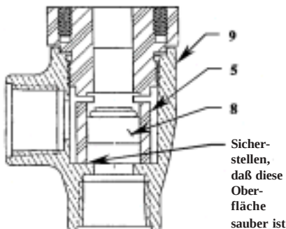
B-0968/B-0969 Querschnitt
