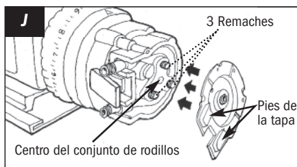
Alinee la tapa del cabezal como se muestra
